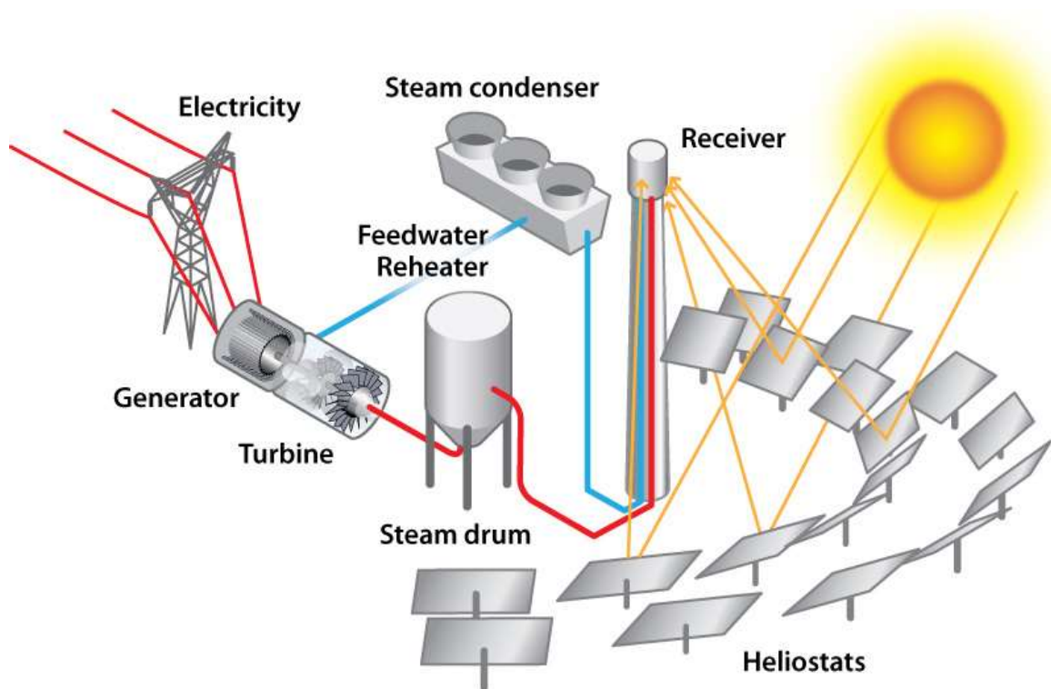
塔式光热太阳能系统示意图（源自 https://www.energy.gov/eere/solar/articles/concentrating-solar-power-tower-plant-illustration ）
